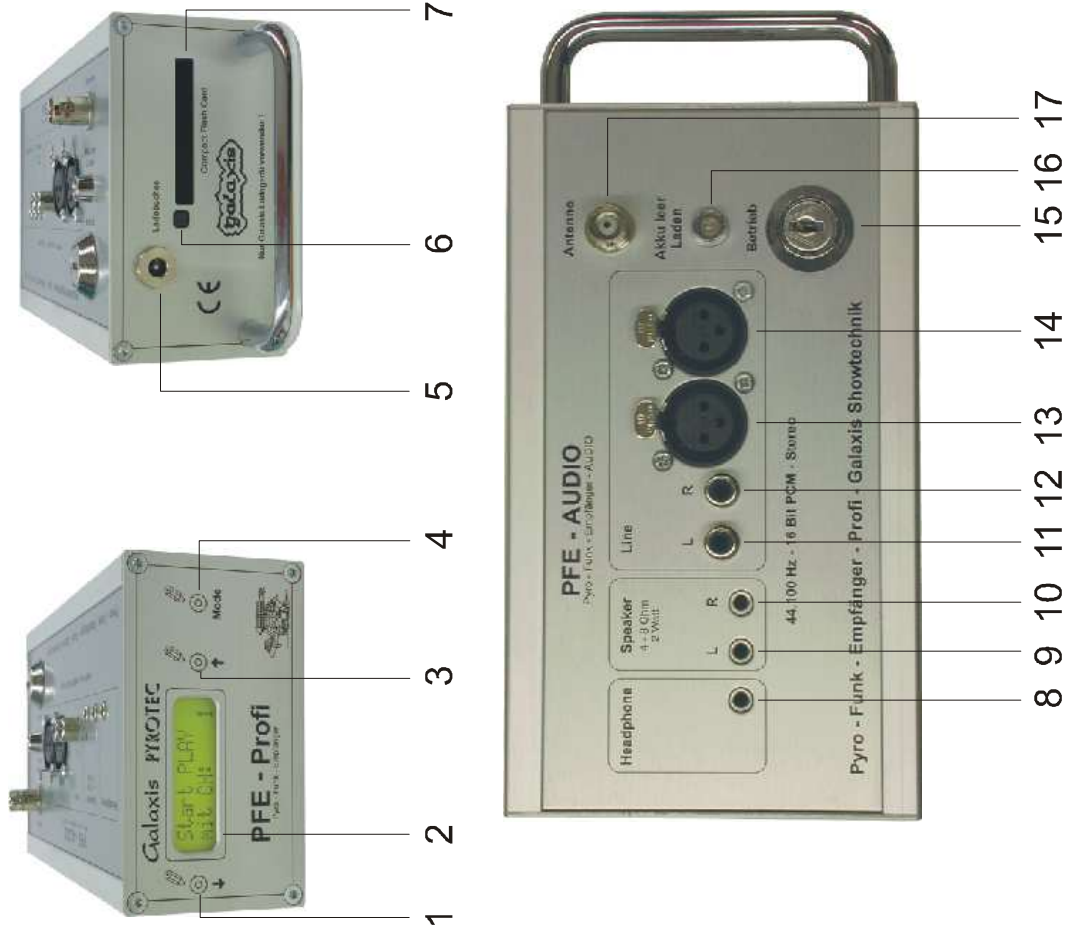
Geräteansicht mit Bedien- und Anzeigeelementen
